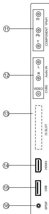
Боковая панель разъемов
